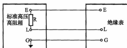
图1 检测基本误差接线图
