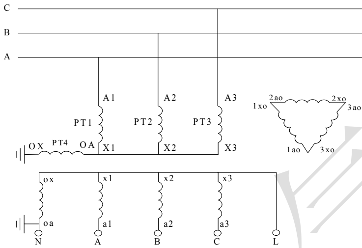
图 7 4PT 接线方式一
