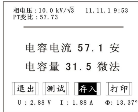
图 18 存入测量数据
