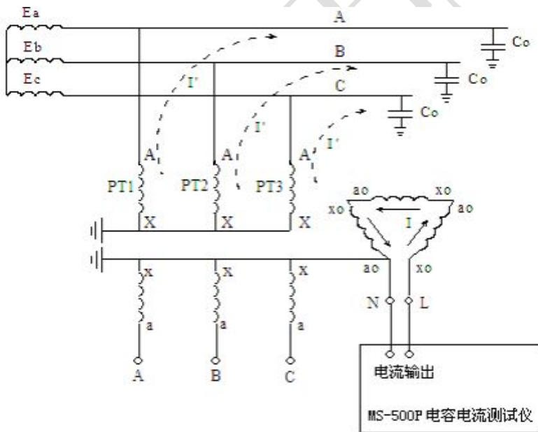
图 2 测量原理图
