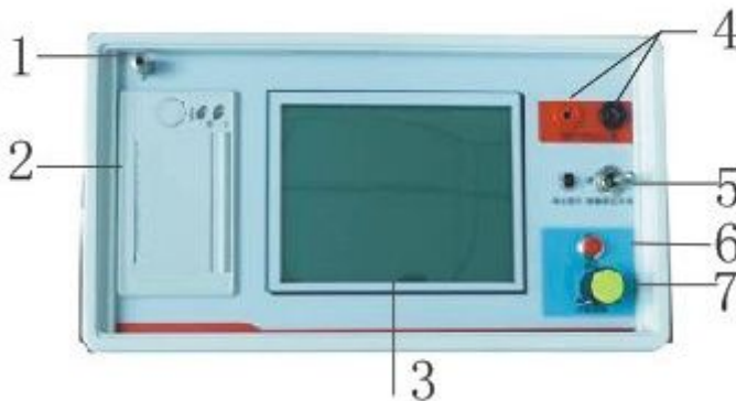
图 1 面板介绍
