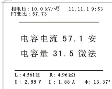
图 17 测量结果显示
